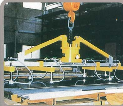
フコク(株) ERDバキュームリフト
